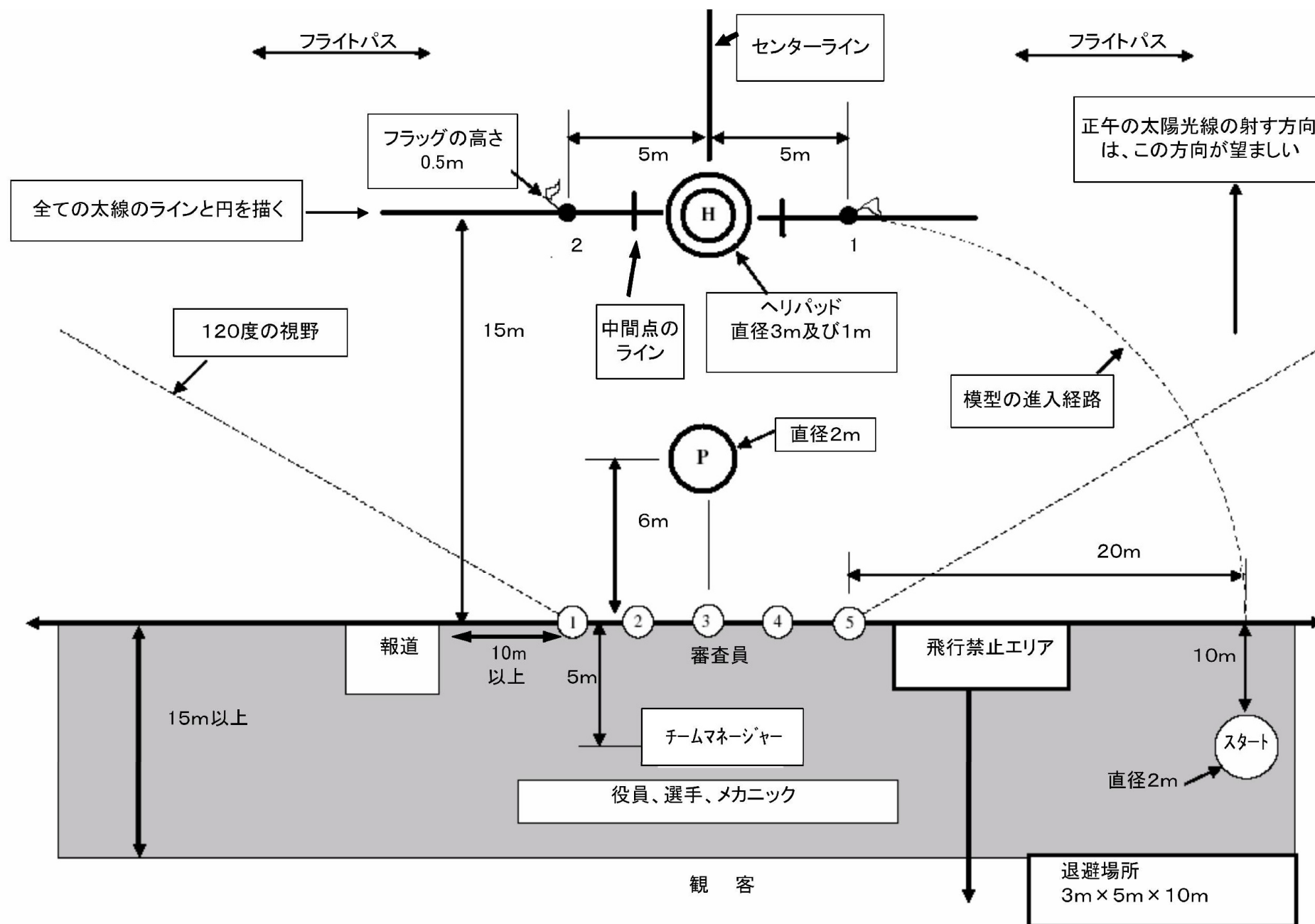
図5.4.A F3C コンテストエリア・レイアウト
